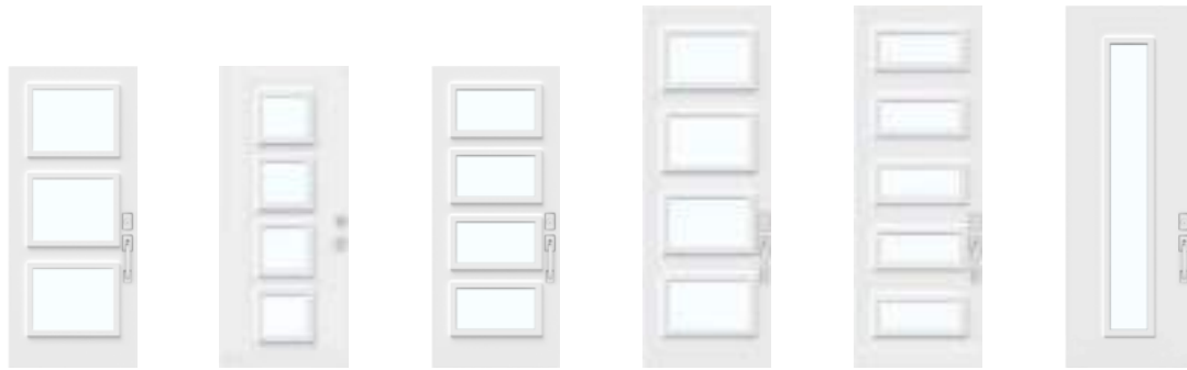
22"×17" 12"×12" 22"×12" 22"×14 1/16" 22"×9" 10 15/16"×76 1/16"
